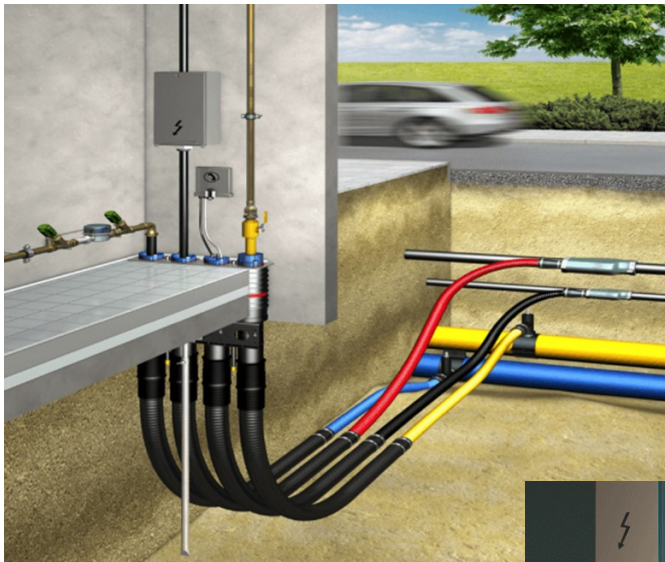
Mehrsparteneinführung Haus ohne Keller
