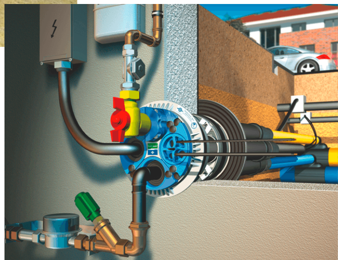
Mehrsparteneinführung Haus mit Keller
