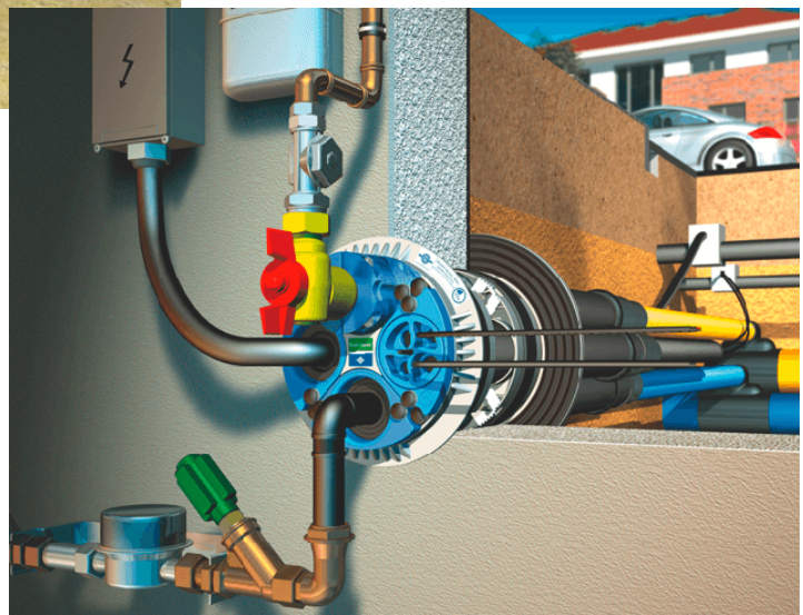
Mehrsparteneinführung Haus mit Keller
